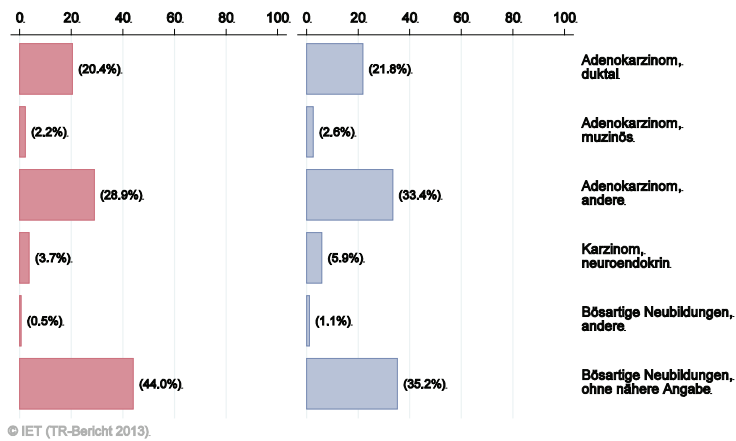
Abbildung 71: Histologieverteilung Pankreaskarzinom 2004–2013
