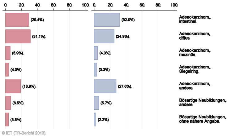
Abbildung 42: Histologieverteilung Magenkarzinom 2004–2013
